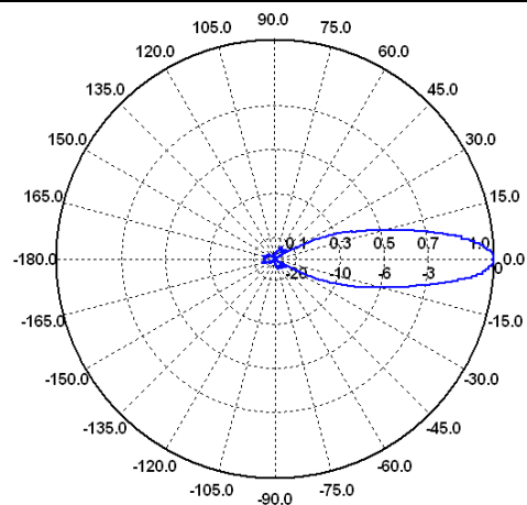
H-Ebene / H-Plane 15 GHz
